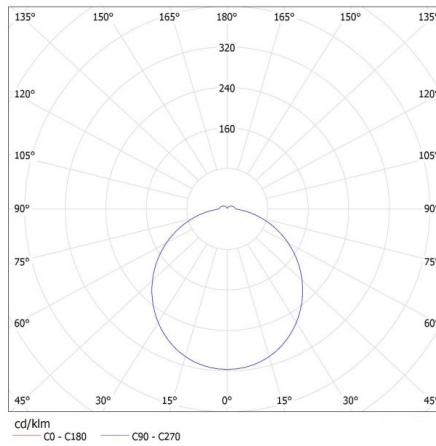
KANLUX S.A. (kat 26444) VARSO LED 24W-WW-O / Krzywa rozsytu światła (biegunowo)
