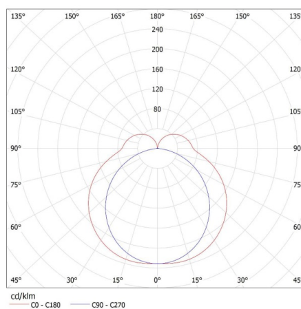
KANLUX S.A. (kat 27118) TP SLIM TW LED 50W-NW / LDC (Polar)
