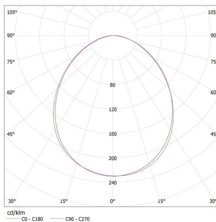
KANLUX S.A. (kat 27410) ALIN 4LED 1X60-W + Miledo / LDC (Polar)
