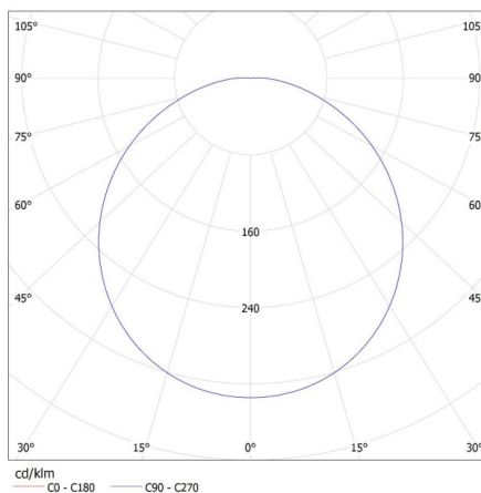
KANLUX S.A. (kat 32530) DROMI LED EL-1 7W-GR / LDC (Polar)
