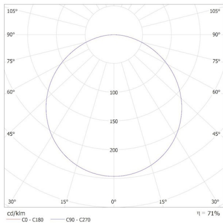
KANLUX S.A. (kat 33178) BLINGO TN 24-28W 6060 NW (28) / Krzywa rozsyłu światła (biegunowo)
