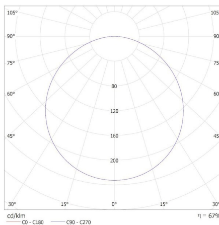
KANLUX S.A. (kat 33178) BLINGO TN 24-28W 6060 NW (24) / Krzywa rozsyłu światła (biegunowo)
