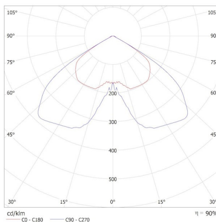
KANLUX S.A. (kat 36435) PARCOLI 30-50W CCT G_0st / Krzywa rozsyłu światła (biegunowo)
