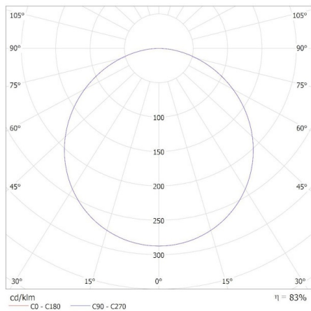
KANLUX S.A. (kat 37172) BLINGO 34W 4080 60CW / Krzywa rozsytu światła (biegunowo)
