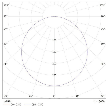
KANLUX S.A. (kat 37178) BLINGO 24W 4320 60NW / Krzywa rozsytu światła (biegunowo)
