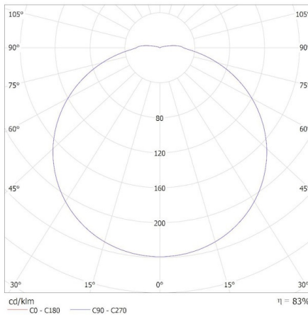
KANLUX S.A. (kat 37290) IPER LED 10W-NW-O / Krzywa rozsytu światła (biegunowo)
