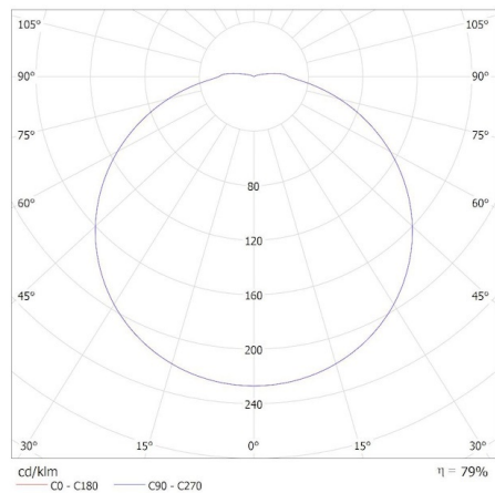
KANLUX S.A. (kat 37291) IPER LED 19W-NW-O / Krzywa rozsytu światła (biegunowo)
