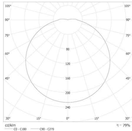
KANLUX S.A. (kat 37299) IPER LED 19W-NW-O-SE / Krzywa rozsytu światła (biegunowo)
