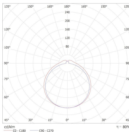
KANLUX S.A. (kat 38796) LINCEA 30-45W 12 CCT 3000K / Krzywa rozsyłu światła (biegunowo)
