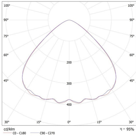
KANLUX S.A. (kat 27159 + 38128) HB PRO STRONG 200W-NW + LENS 60D / Krzywa rozsyłu światła (biegunowo)
