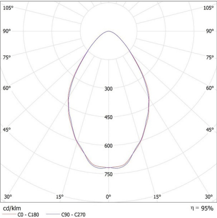
KANLUX S.A. (kat 27159 + 38129) HB PRO STRONG 200W-NW + LENS 120D / Krzywa rozsyłu światła (biegunowo)
