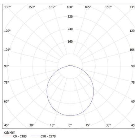
KANLUX S.A. (kat 26444) VARSO LED 24W-WW-O / Krzywa rozsyłu światła (biegunowo)
