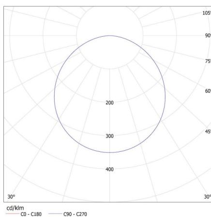
KANLUX S.A. (kat 27212) KANTI V2LED 12W-NW-SN / LDC (Polar)
