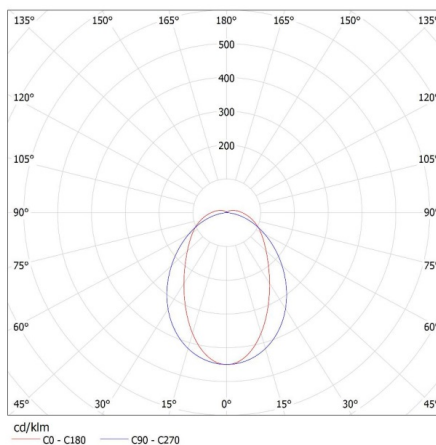
KANLUX S.A. (kat 28661) FT1500 55W-840-INT / LDC (Polar)
