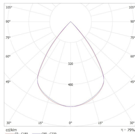
KANLUX S.A. (kat 33921) AL-SH-NW-RST-B-NT / Krzywa rozsyłu światła (biegunowo)
