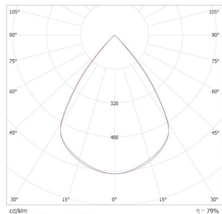
KANLUX S.A. (kat 33992) AL-ML-NW-RST-B-NT / Krzywa rozsyłu światła (biegunowo)
