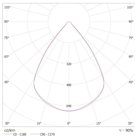
KANLUX S.A. (kat 34089) AL-LH-NW-RST-W-NT / Krzywa rozsyłu światła (biegunowo)
