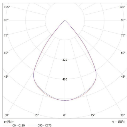
KANLUX S.A. (kat 34101) AL-LH-NW-RST-B-NT / Krzywa rozsyłu światła (biegunowo)
