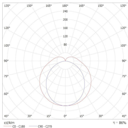
KANLUX S.A. (kat 36652) AKVO IP44 15W-NW-C S / Krzywa rozsytu światła (biegunowo)
