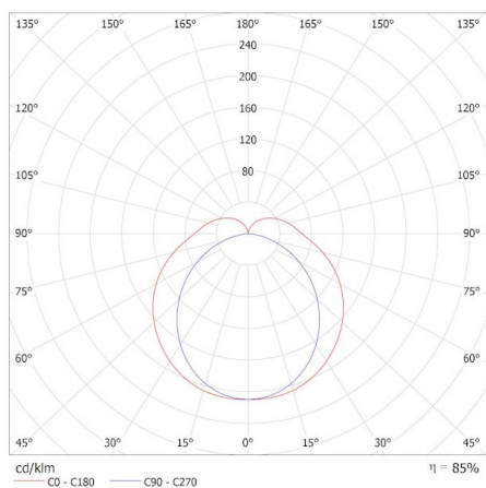
KANLUX S.A. (kat 36655) AKVO IP44 20W-NW-C S / Krzywa rozsyłu światła (biegunowo)
