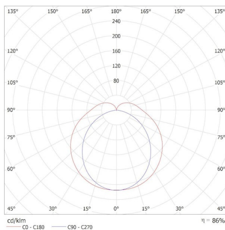
KANLUX S.A. (kat 36660) AKVO IP44 15W-NW-B / Krzywa rozsytu światła (biegunowo)
