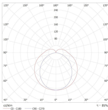
KANLUX S.A. (kat 36663) AKVO IP44 20W-NW-B / Krzywa rozsytu światła (biegunowo)
