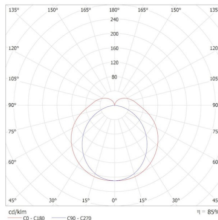
KANLUX S.A. (kat 36664) AKVO IP44 20W-NW-C / Krzywa rozsyłu światła (biegunowo)
