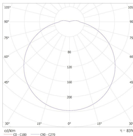
KANLUX S.A. (kat 37302) IPER LED 10W-NW-L- SE / Krzywa rozsytu światła (biegunowo)
