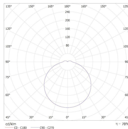
KANLUX S.A. (kat 37304) IPER LED 26W-NW-L-SE / Krzywa rozsyłu światła (biegunowo)
