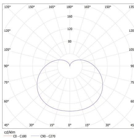
KANLUX S.A. (kat 27276) IQ-LED A60 10,5W-WW / LDC (Polar)
