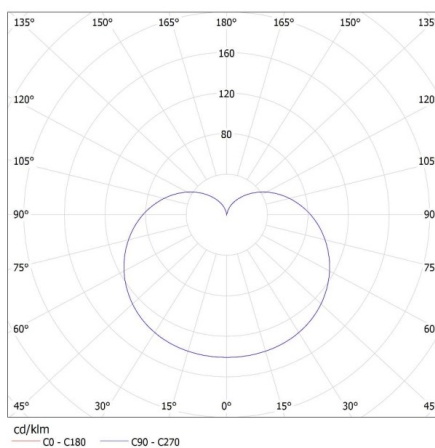
KANLUX S.A. (kat 27307) IQ-LED G45E14 7,5W-NW / LDC (Polar)
