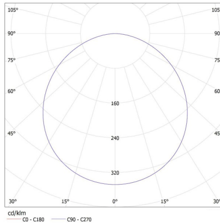
KANLUX S.A. (kat 28949) CARSA V2LED 18W-NW-W / LDC (Polar) Luminaire: KANLUX S.A. (kat 28949) CARSA V2LED 18W-NW-W Lamps: 1 x CARSA V2LED 18W-NW-W
