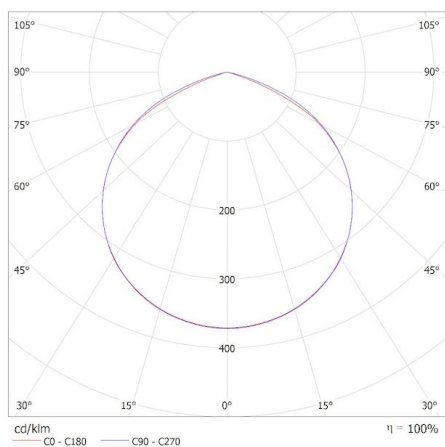
KANLUX S.A. (kat 29225) STATO HI LED 50W-B / Krzywa rozsyłu światła (biegunowo)
