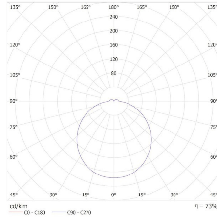
MILED0 (kat 31490) TURA LED 15W-NW-O-B / Krzywa rozsytu światła (biegunowo)
