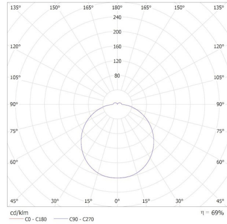
MILED0 (kat 31491) TURA LED 24W-NW-O-B / Krzywa rozsytu światła (biegunowo)
