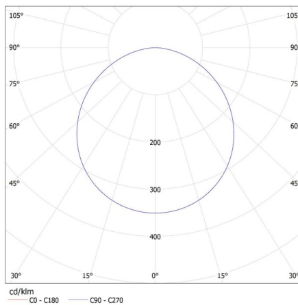
KANLUX S.A. (kat 33551) KANTI V2LED 12W-WW-B / LDC (Polar)
