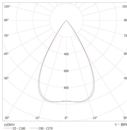
KANLUX S.A. (kat 37114) HR-LH-WW-W-RM / Krzywa rozsyłu światła (biegunowo)
