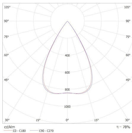
KANLUX S.A. (kat 37117) HR-MM-WW-B-RM / Krzywa rozsyłu światła (biegunowo)
