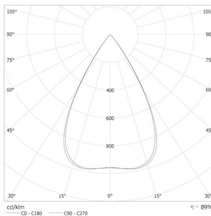
KANLUX S.A. (kat 37139) HR-MH-NW-W-RM / Krzywa rozsyłu światła (biegunowo)
