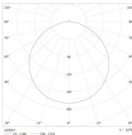
KANLUX S.A. (kat 37317) NIFU LED17,8W NW W_BR / Krzywa rozsyłu światła (biegunowo)
