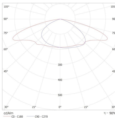
KANLUX S.A. (kat 39283) PRO-S M 85W NW / Krzywa rozsyłu światła (biegunowo)
