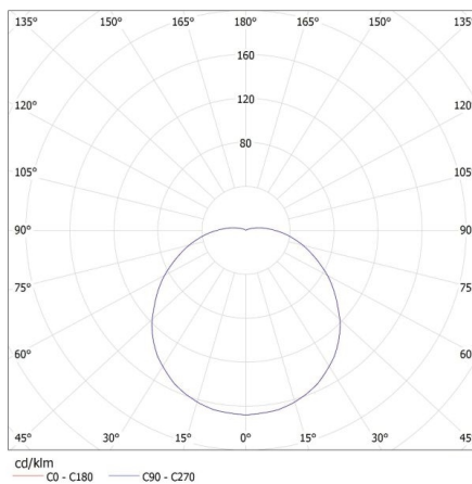
KANLUX S.A. (kat 7015) MARC DL-60 / Krzywa rozsytu światła (biegunowo)
