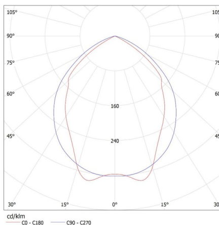
KANLUX S.A. (kat 22671) NOTUS 4LED 418 NT + T8 Miledo / Krzywa rozsyłu światła (biegunowo)
