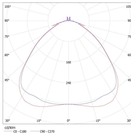
KANLUX S.A. (kat 26033) FULLED GU10-3,3W-WW / Krzywa rozsyłu światła (biegunowo)
