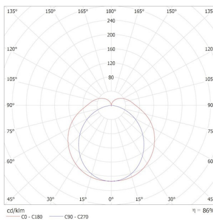
KANLUX S.A. (kat 36665) AKVO IP44 23W-NW-W / Krzywa rozsyłu światła (biegunowo)
