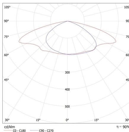
KANLUX S.A. (kat 39292) PRO-S S 25W-ZH NW / Krzywa rozsyłu światła (biegunowo)
