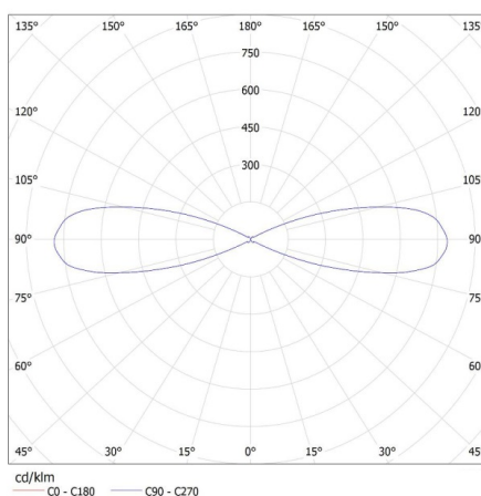
KANLUX S.A. (kat 22443) ZEW EL-235U-GR + IQ-LED ... 7W S3 / LDC (Polar)
