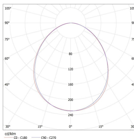
KANLUX S.A. (kat 27411) ALIN 4LED 1X60-B + Miledo / LDC (Polar)
