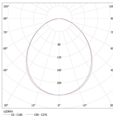
KANLUX S.A. (kat 27411) ALIN 4LED 1X60-B + GLASSv3 / LDC (Polar)
