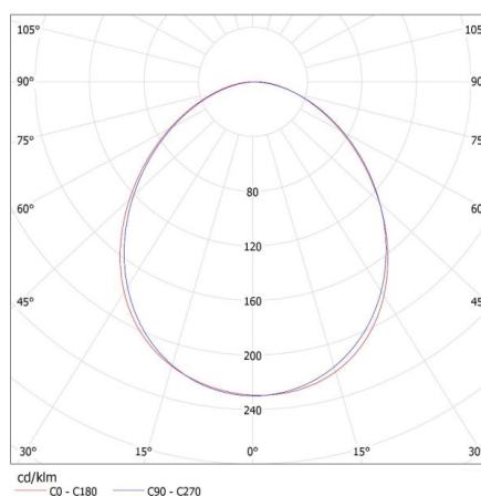
KANLUX S.A. (kat 27422) ALIN 4LED 1X150-W + Miledo / LDC (Polar)
