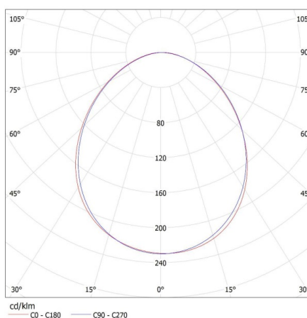
KANLUX S.A. (kat 27424) ALIN 4LED 1X150-SR + Miledo / LDC (Polar)
