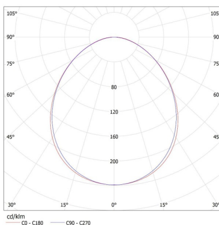
KANLUX S.A. (kat 27424) ALIN 4LED 1X150-SR + GLASSv3 / LDC (Polar)
