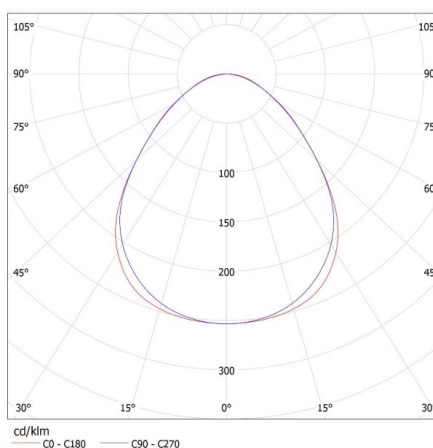
KANLUX S.A. (kat 28447) AL 4LED 120-MPR-B-NT + GLASSv3 / LDC (Polar)
