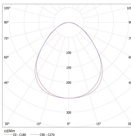
KANLUX S.A. (kat 28448) AL 4LED 120-MPR-SR-NT + GLASSv3 / LDC (Polar)
